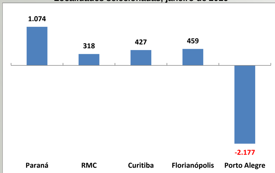
GRÁFICO 2 Saldo do emprego formal celetista Localidades selecionadas, janeiro de 2016
