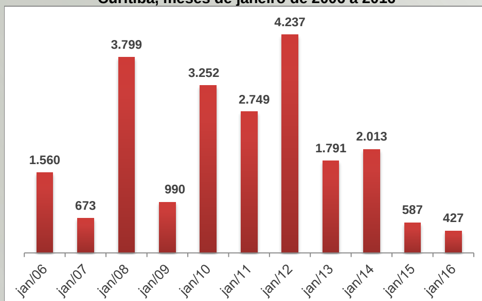
GRÁFICO 1 Saldo do emprego formal celetista Curitiba, meses de janeiro de 2006 a 2016
