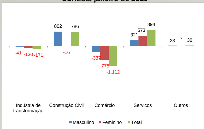
GRÁFICO 3 Saldo do emprego formal celetista por setor de atividade e sexo Curitiba, janeiro de 2016
